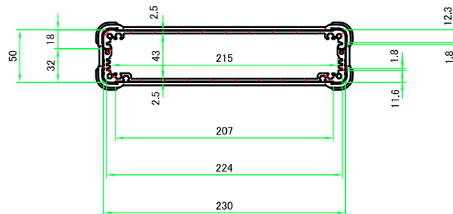
A-A (1:5)
